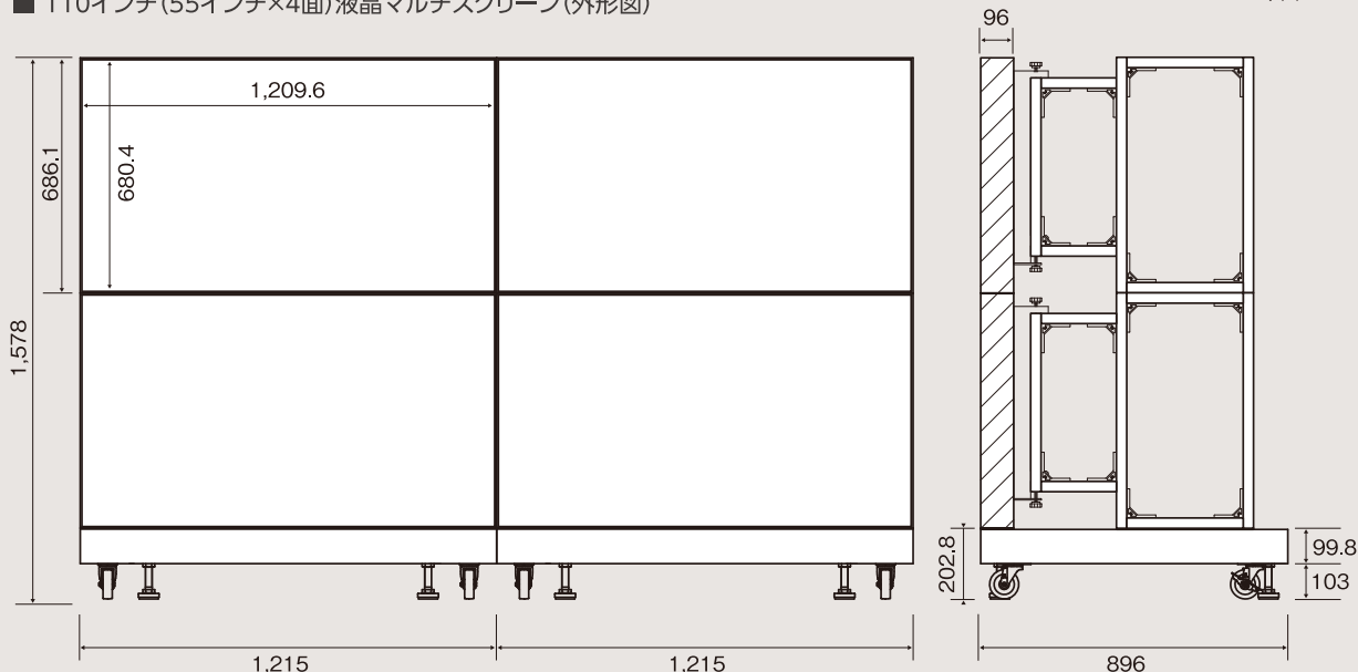
■ 110インチ(55インチ×4面)液晶マルチスクリーン(外形図)
