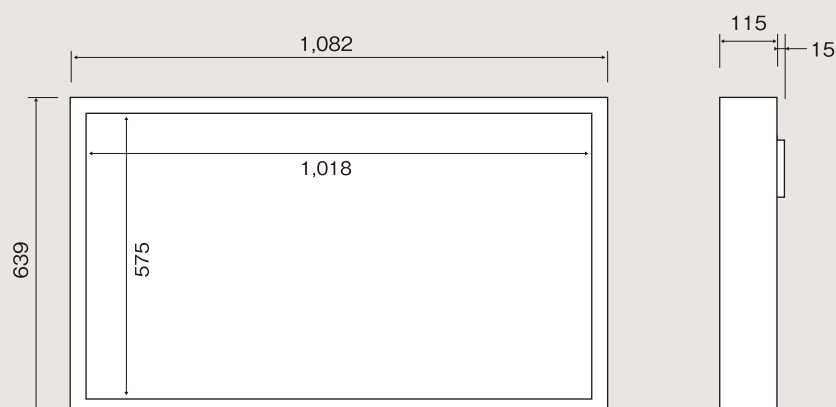
■ 46型・屋外設置全天候型液晶ディスプレイ (外形図)
