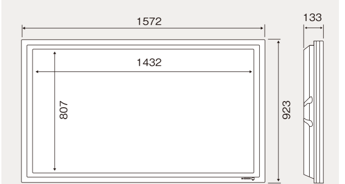
■ 65型液晶ディスプレイ(外形図) (単位:mm)
